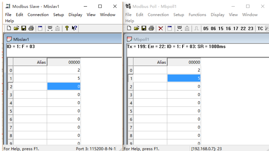
图37 Modbusrtu 转 Modbus tcp 转换结果
