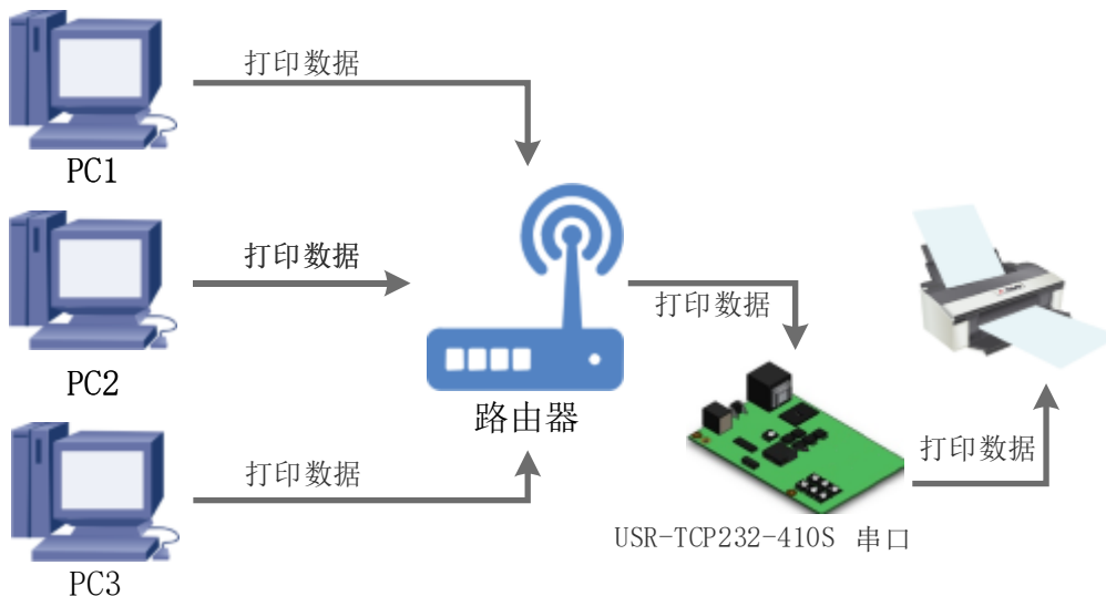
图50 网络打印功能
