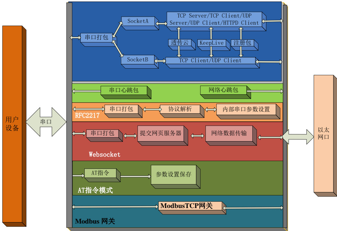
图1 410s 功能框图
