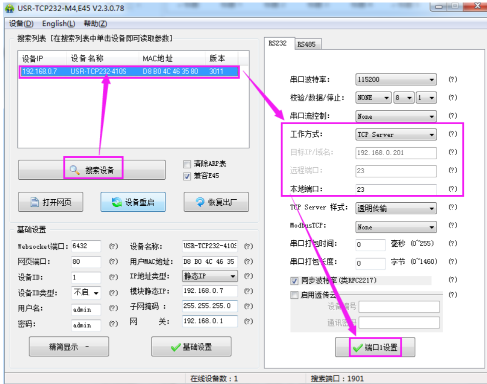
图12 TCP Server 软件设置图
