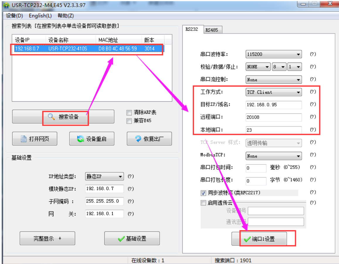
图8 TCP Client 软件设置
