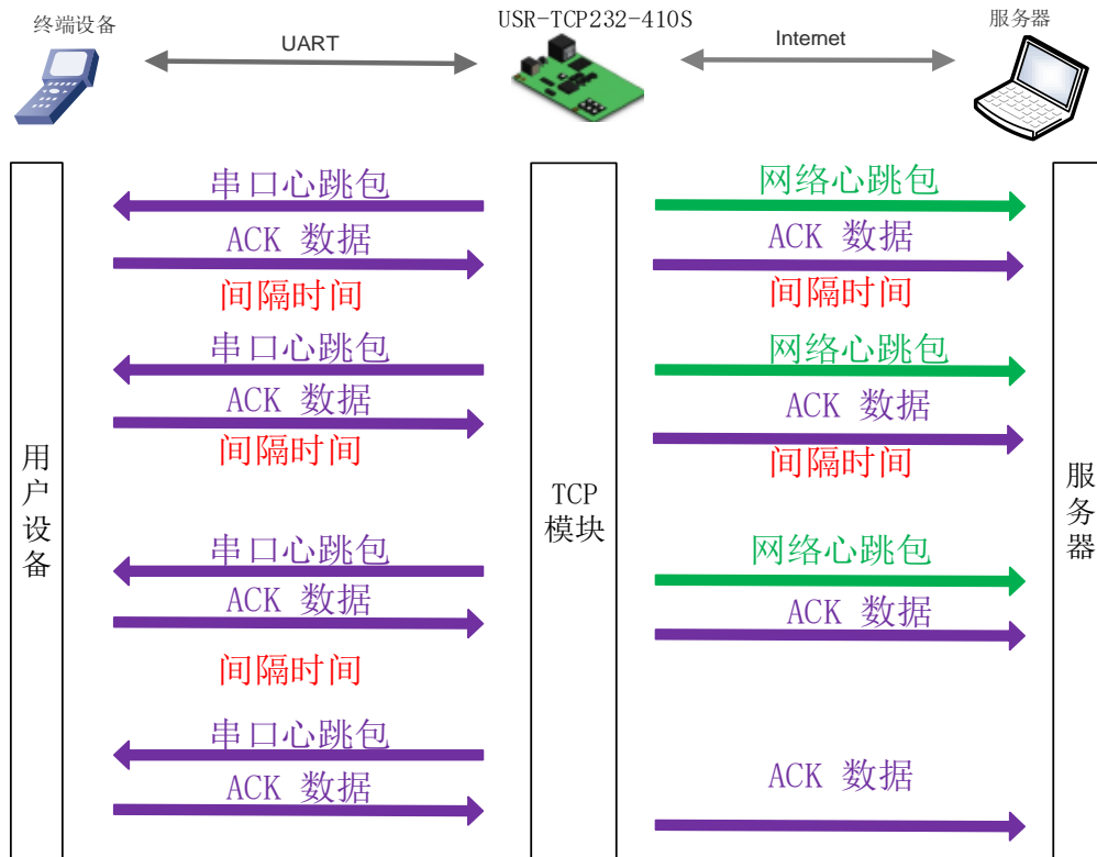
图32 心跳包功能示意图
