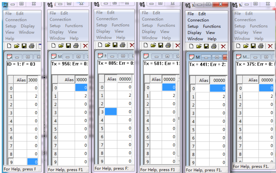
图44 Modbus 轮询测试截图
