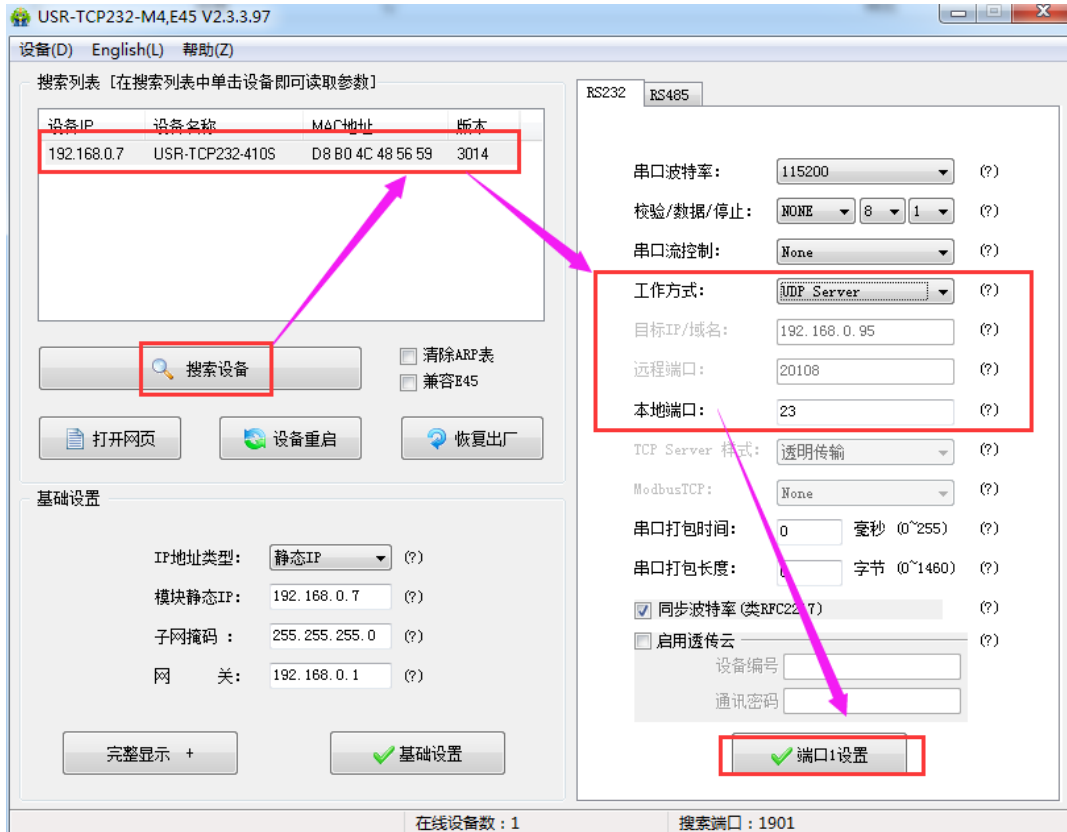
图20 UDP Server 软件设置图
