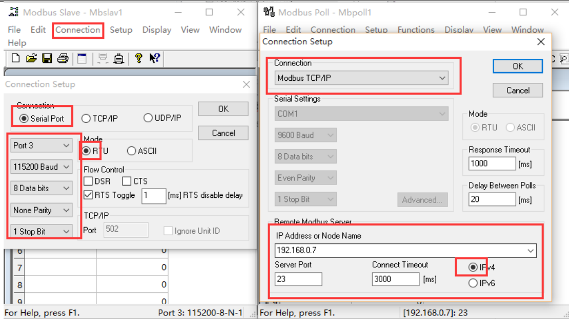
图36 Modbusrtu 转 Modbus tcp 软件设置截图
