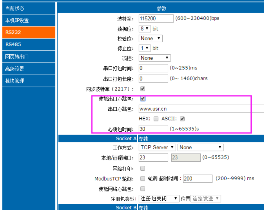
图38 Modbusrtu 主动查询设置截图
