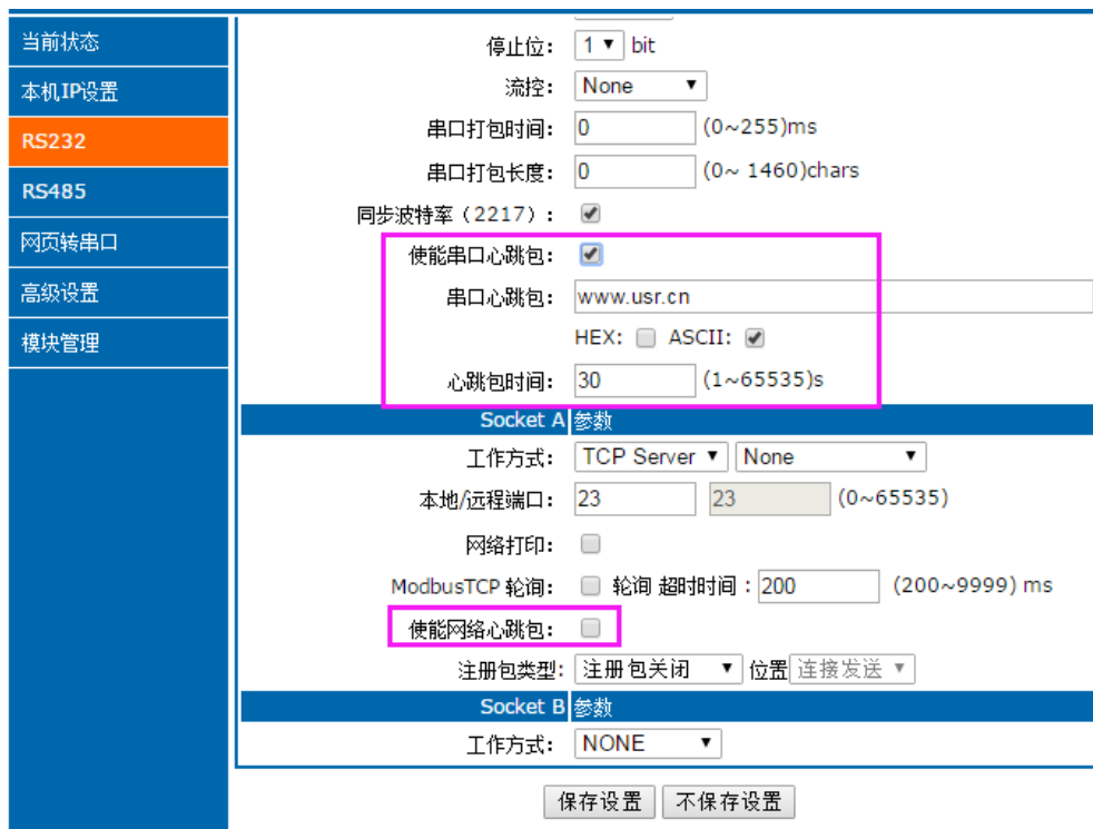
图33 心跳包功能设置
