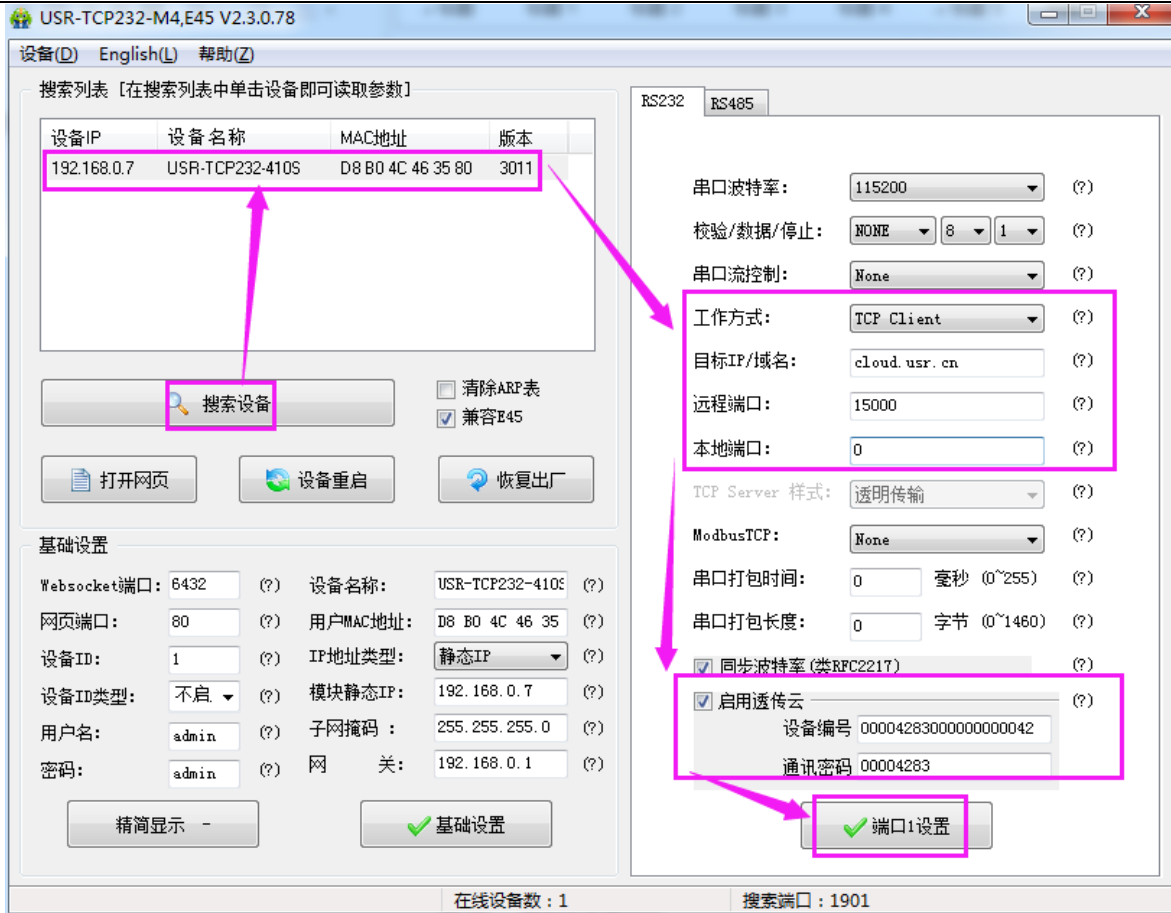
图49 透传云功能设置
