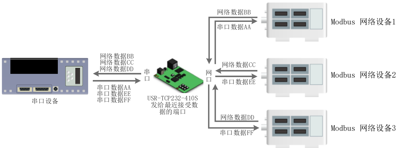
图41 Modbus TCP
