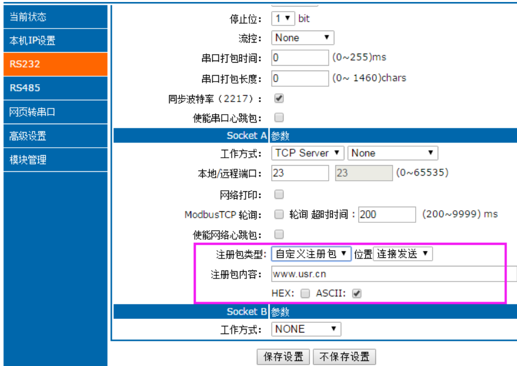
图47 注册包功能
