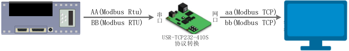
图34 Modbus TCP
