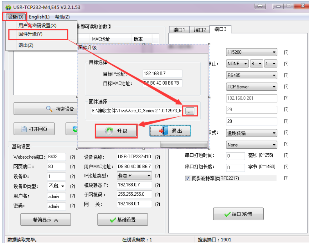
图5 选择固件
