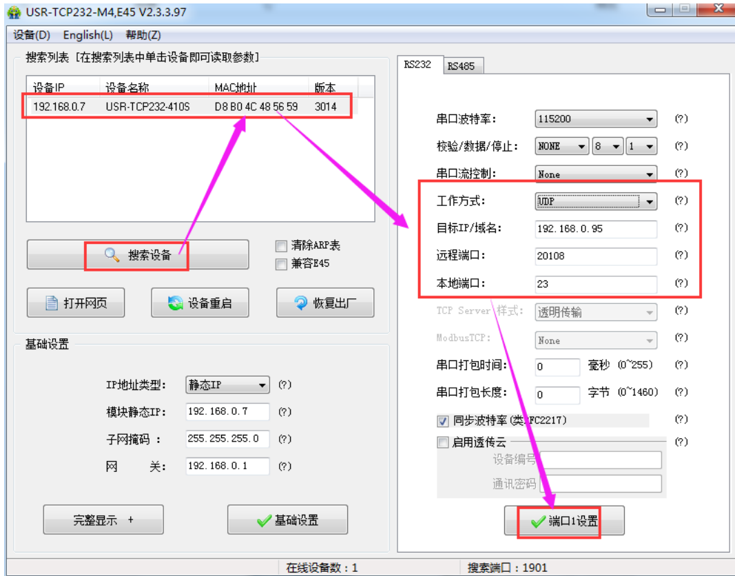
图16 UDP Client 软件设置
