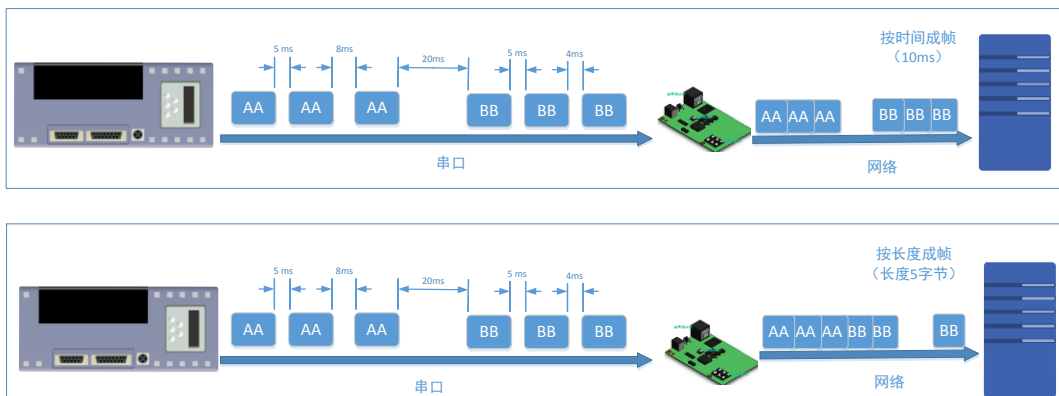
图30 串口成帧说明
