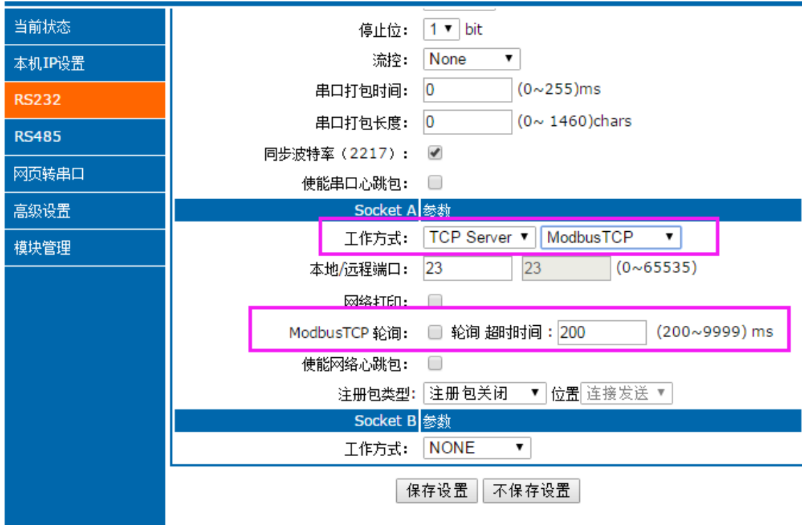
图42 Modbus 轮询网页设置截图
