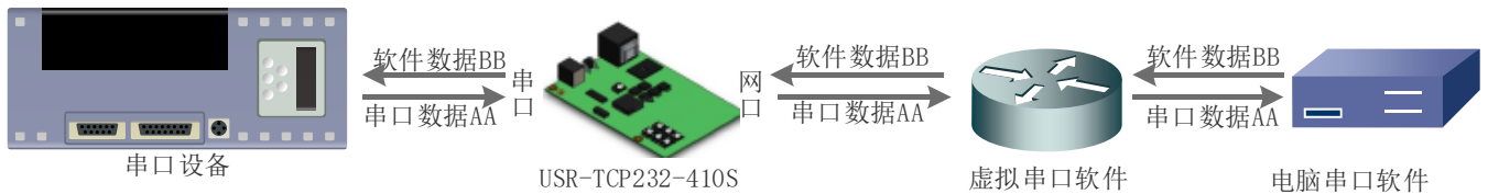
图28 VCOM 应用介绍
