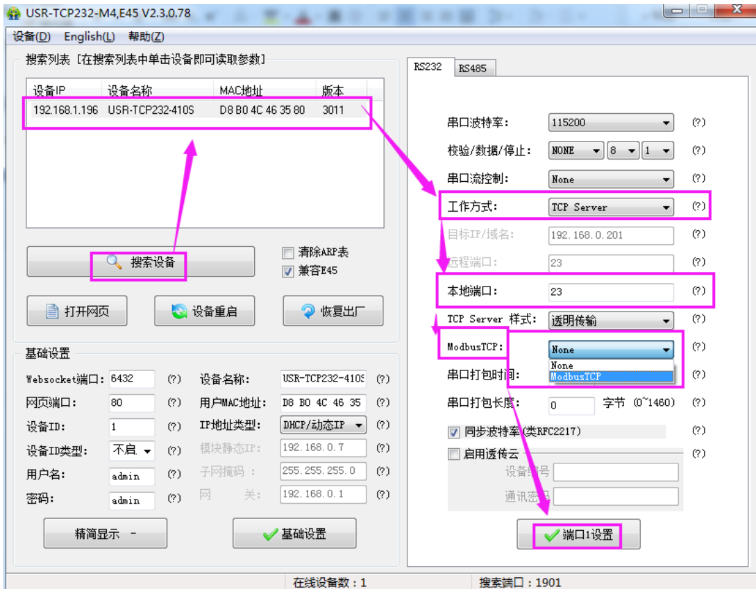
图35 Modbusrtu 转 Modbus tcp
