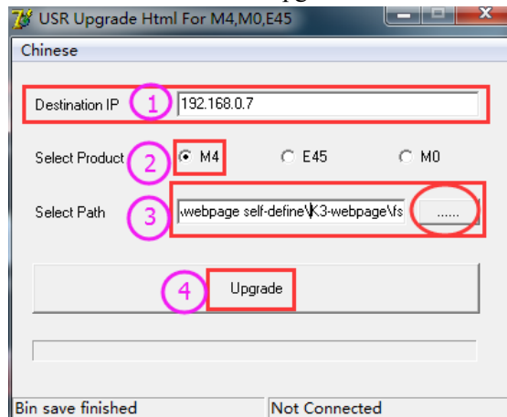
图57 网页升级固件方法截图
