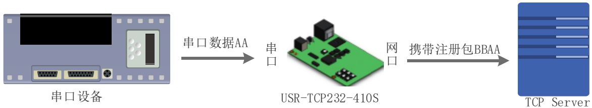
图46 数据携带注册包
