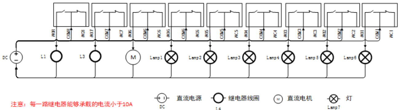
图 20 DO 输出接线图
