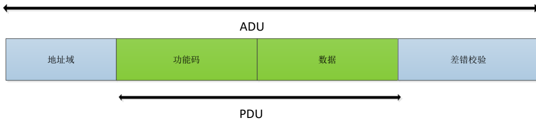
图 39 Modbus RTU 帧
