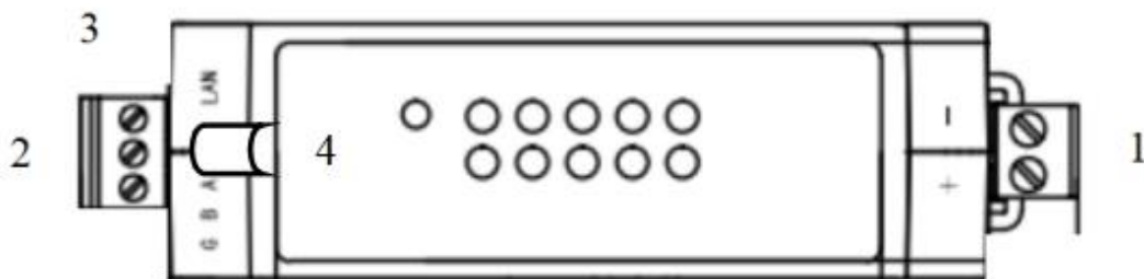
图 1 USR-DR404 串口服务器接口定义
