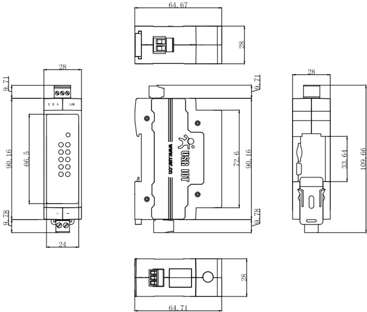
图3 USR-DR404 尺寸图
